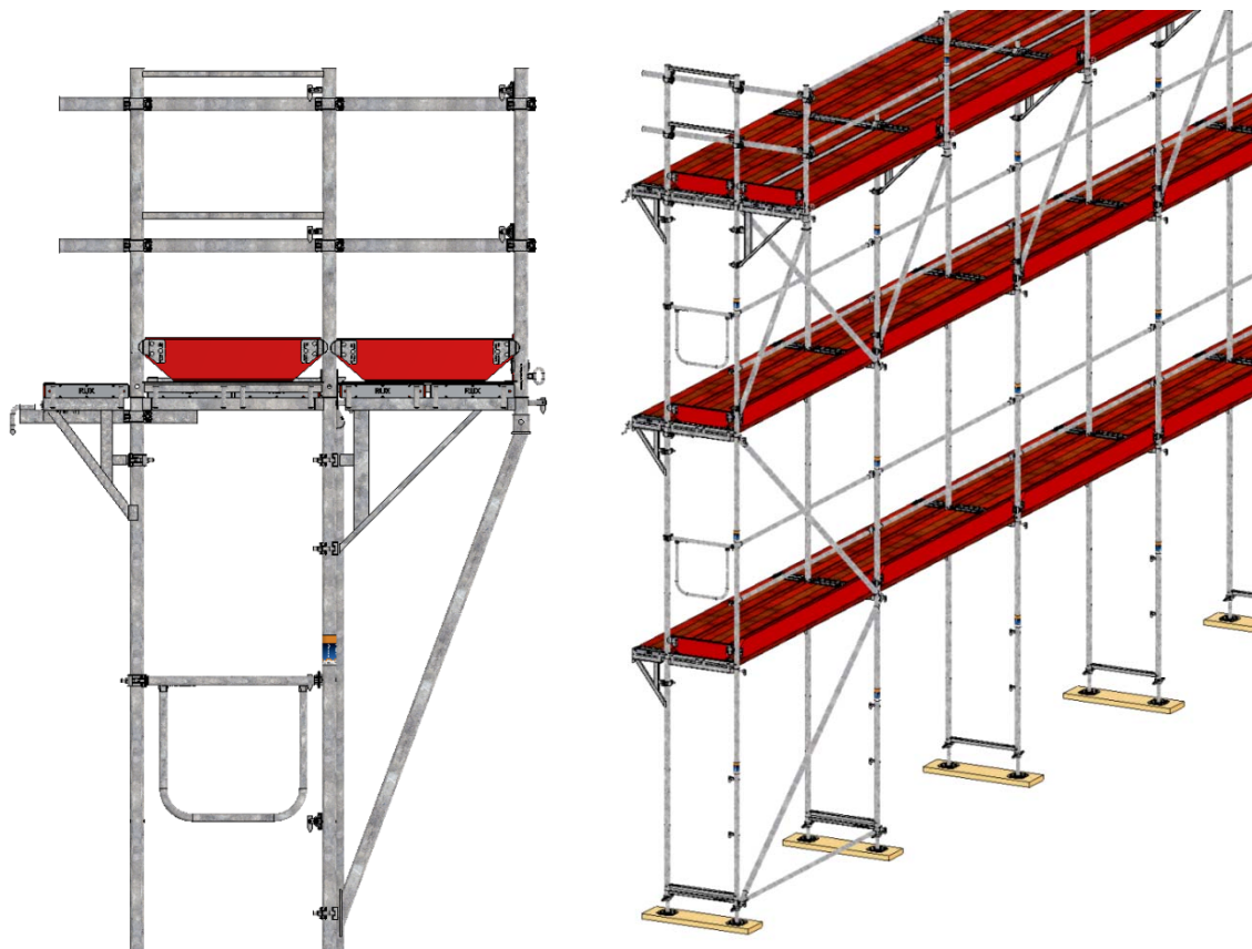
Bild 52: Gerüst mit zweibohlgiger Verbreiterungskonsolen außen und Abfangstrebe
