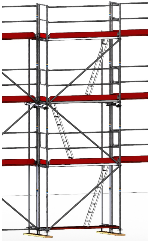
Bild 48: Vorgestellter Leiteraufstieg.
