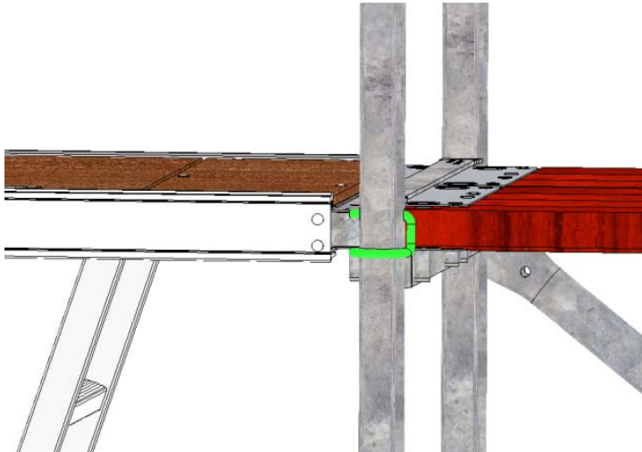
Bild 32: Eingesteckter Fallstecker.
