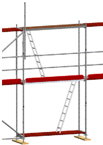
Bild 26: Montage des ersten MSG-Pfostens.
