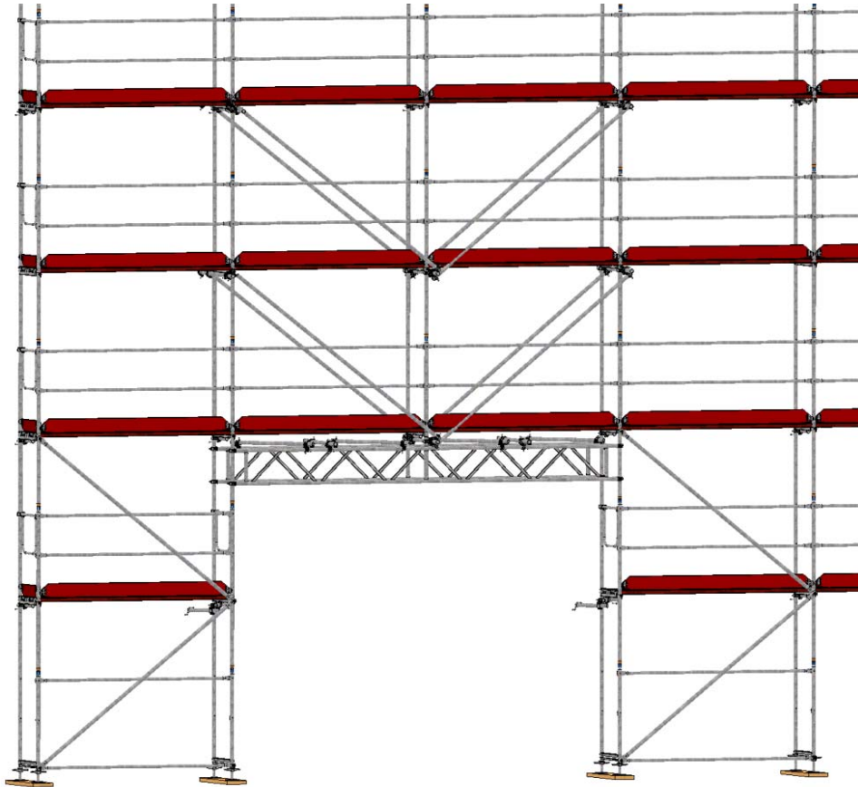
Bild 54: Überbrückung
