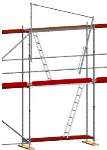
Bild 27: Einhängen des MSG-Geländers und zweiten MSG-Pfosten koppeln.
