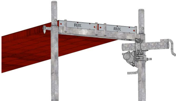
Bild 38: V-Halter, Grundkonfiguration
